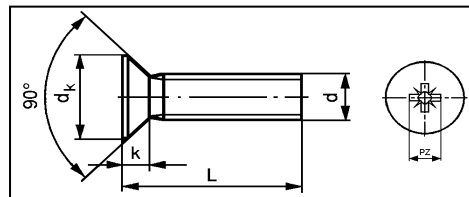
DIN 965
