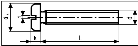
DIN 85
