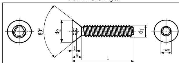
Torx horonnyal
