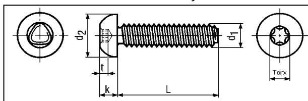
Torx horonnyal
