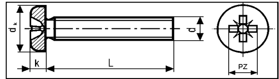
DIN 7985
